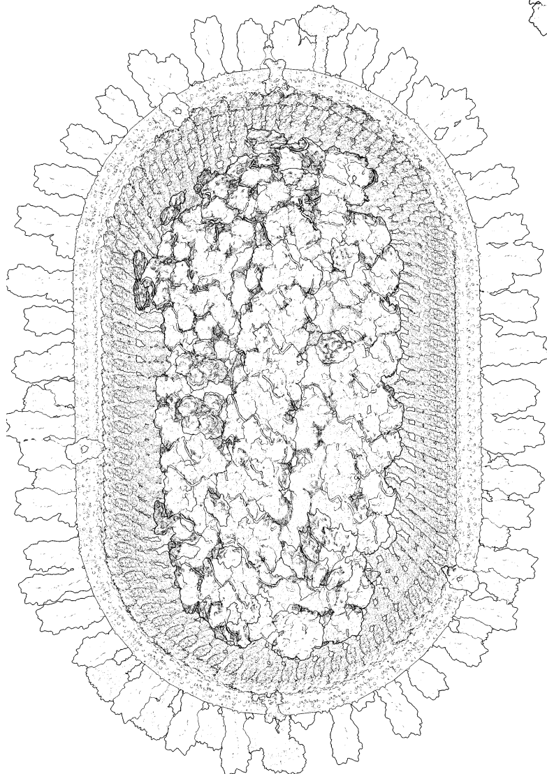
vRNA
